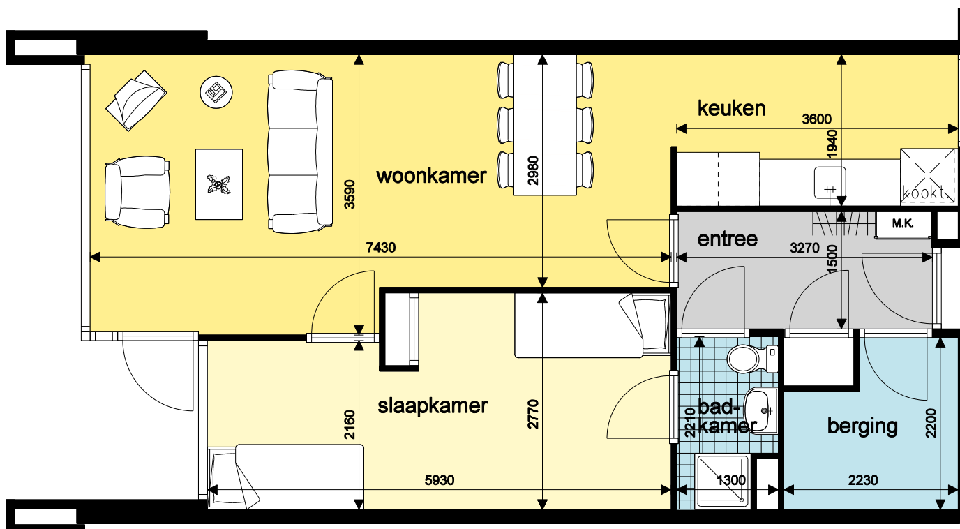
Plattegrond appartement in twee lagen
