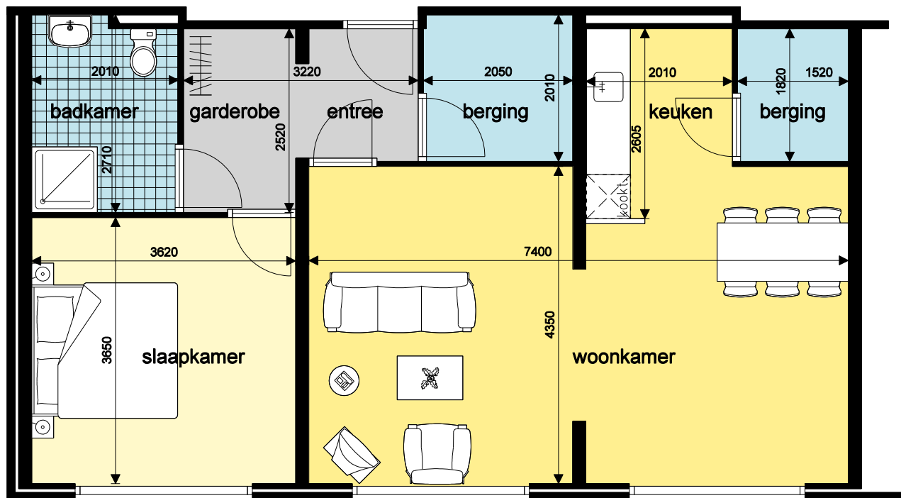
Plattegrond appartement in hoogbouw
